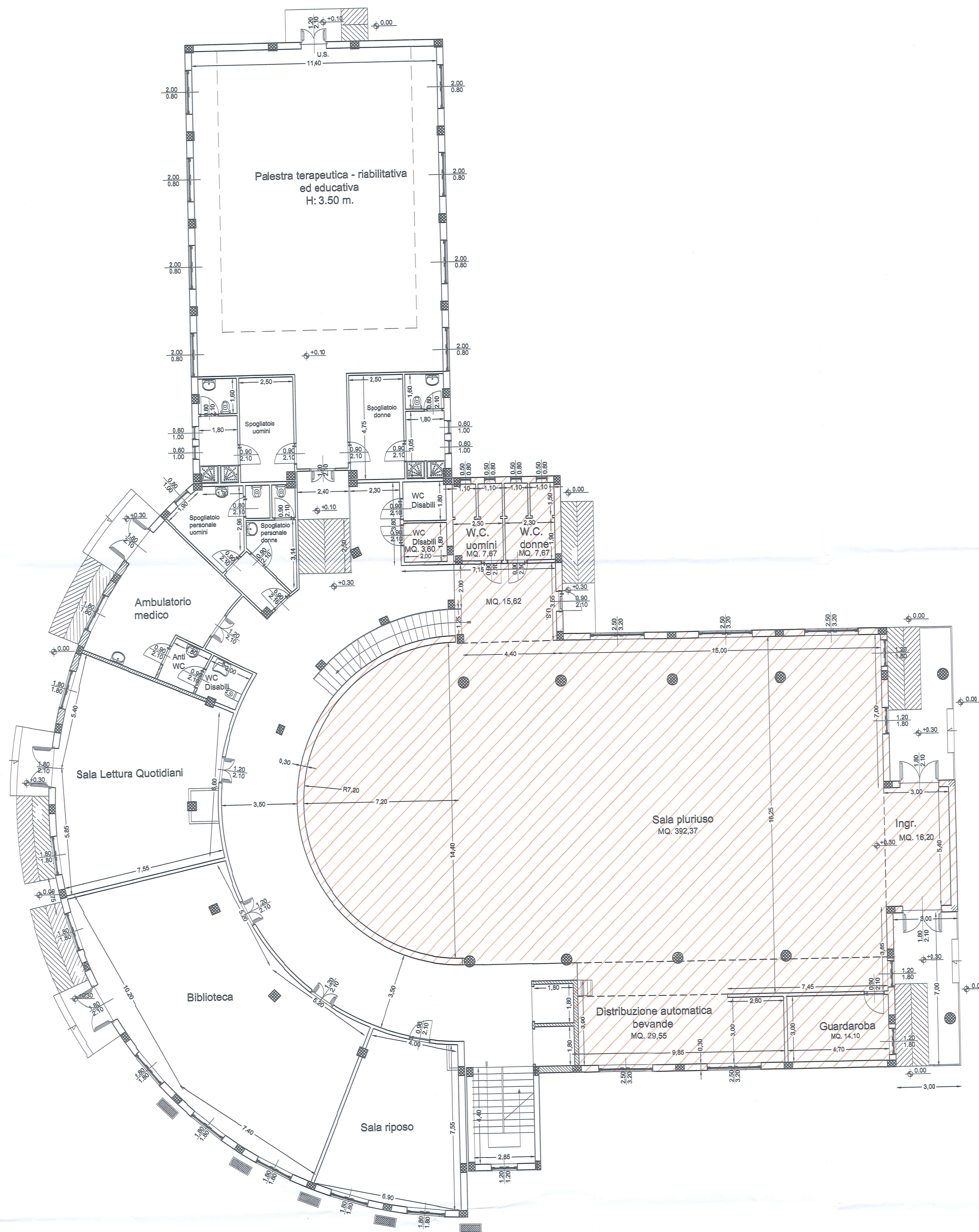
PIANTA PIANO TERRA
