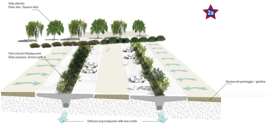
IMMAGINE 4 • SEZIONE PARCHEGGIO ECOLOGICO
